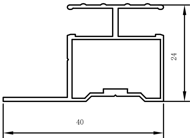
Dørramme profil
