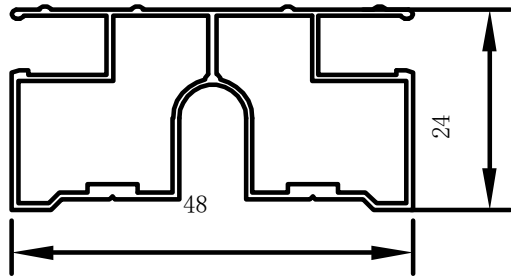
Tag profil
