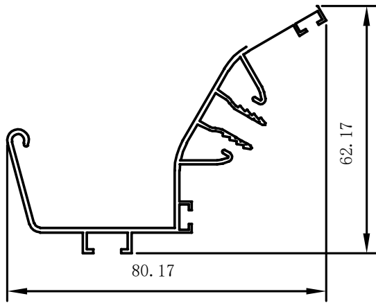
Tagrende profil
