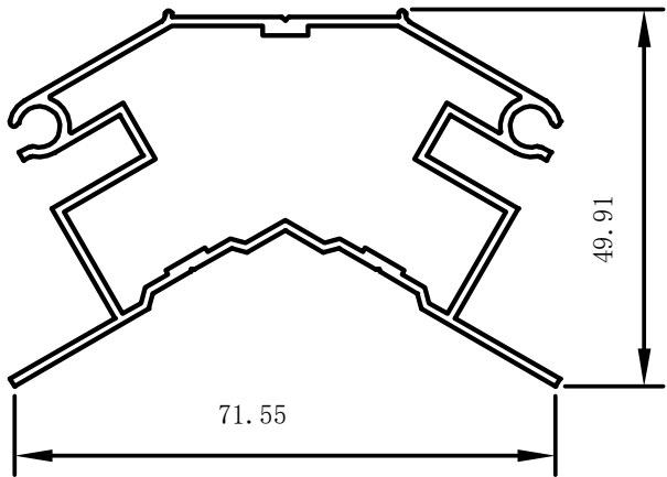
Tagryg profil
